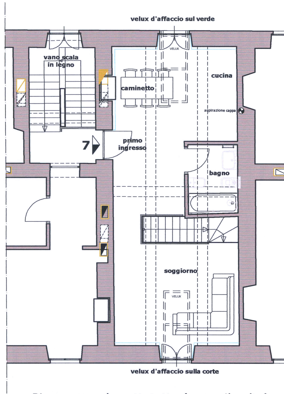
Piano secondo sottotetto (sopra il volto)
