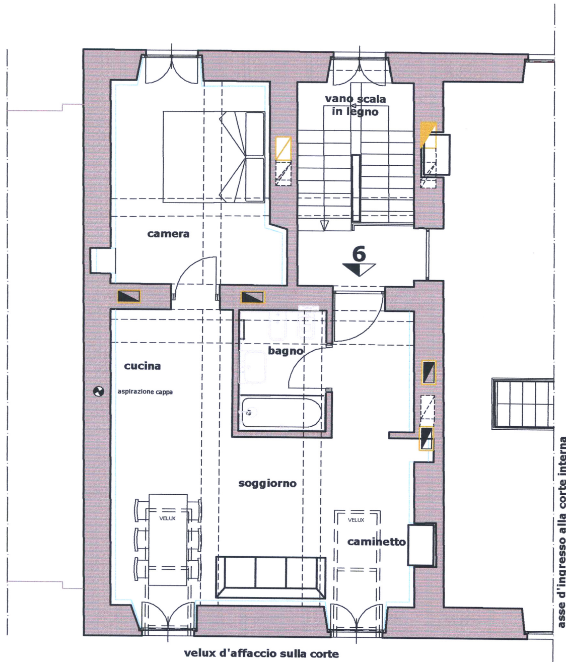
Piano secondo sottotetto
